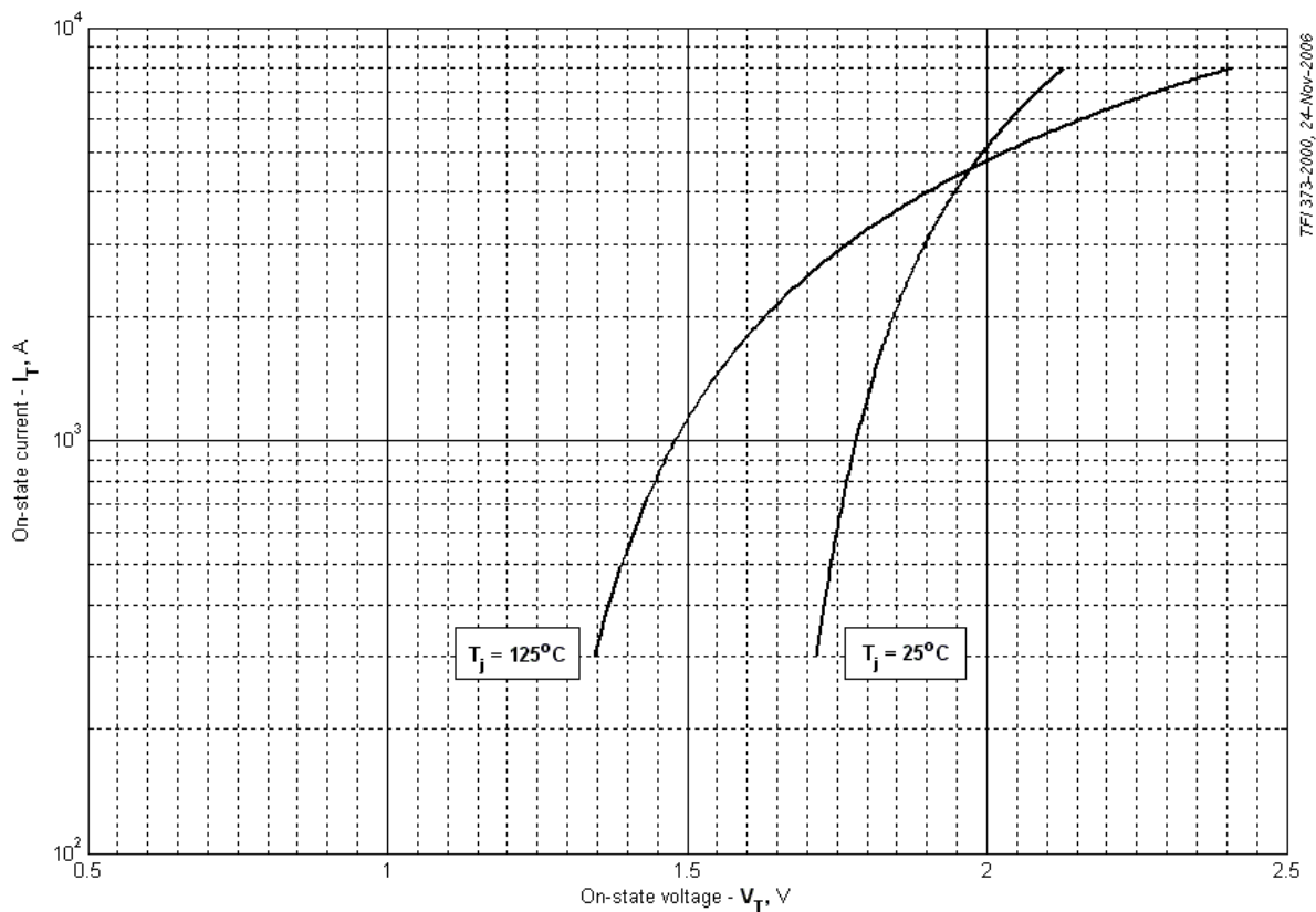
Рис. 1 – Вольт - амперная характеристика в открытом состоянии
