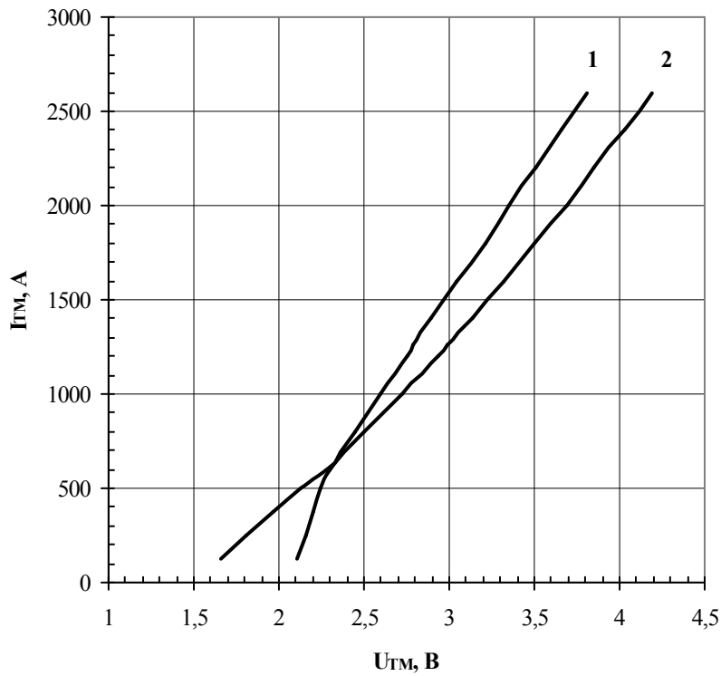
Рис.1 – Предельная вольт-амперная характеристика. 1 – T_j = 25^\circ\text{C} 2 – T_j = 125^\circ\text{C}
