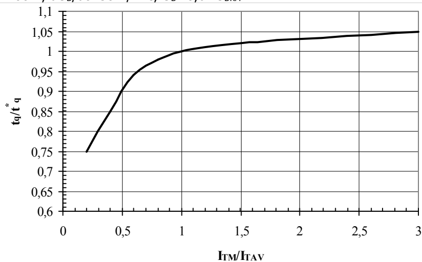
Рис. 28 – Зависимость времени выключения t_q от среднего тока в открытом состоянии I_T/I_{TAV} .
