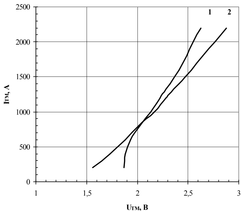
Рис.1 – Предельная вольт-амперная характеристика. 1 – T_j=25\text{ °C} 2 – T_j=125\text{ °C}
