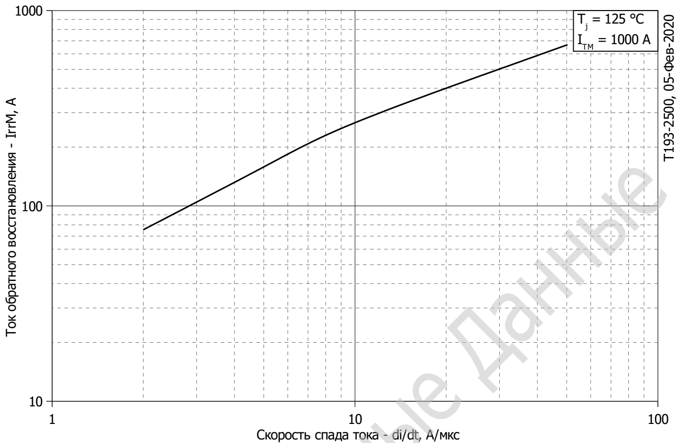
Рис. 7 – Зависимость максимального тока обратного восстановления I_{TM} от скорости спада тока di_R/dt в открытом состоянии
