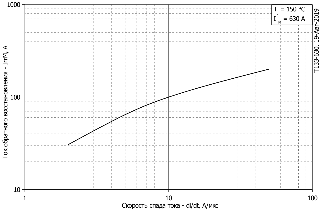
Рис. 5 – Зависимость максимального тока обратного восстановления I тТМ от скорости спада тока di R /dt в открытом состоянии
