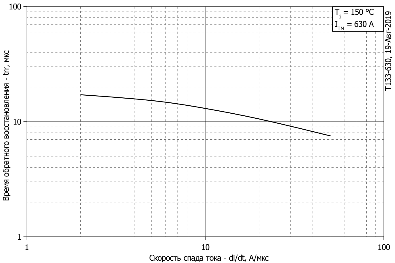
Рис. 6 - Зависимость максимального времени обратного восстановления t тТ от скорости спада тока di R /dt (по ГОСТ 24461, хорда 25%) в открытом состоянии
