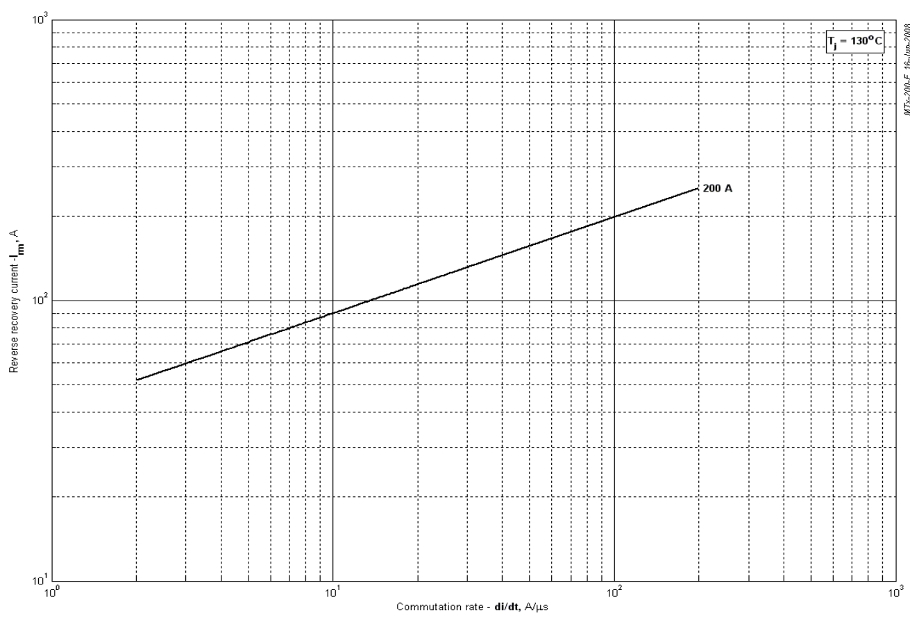
Рис. 7 – Максимальный ток обратного восстановления, I_{rr}
